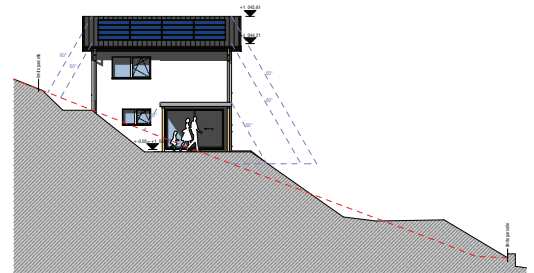
Façade Ouest
