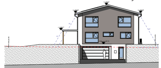
Façade Sud
