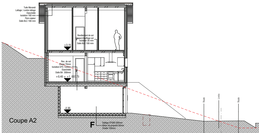
Coupe A2
