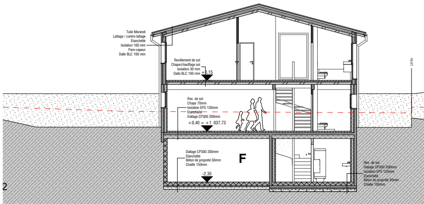
Coupe B2-B2
