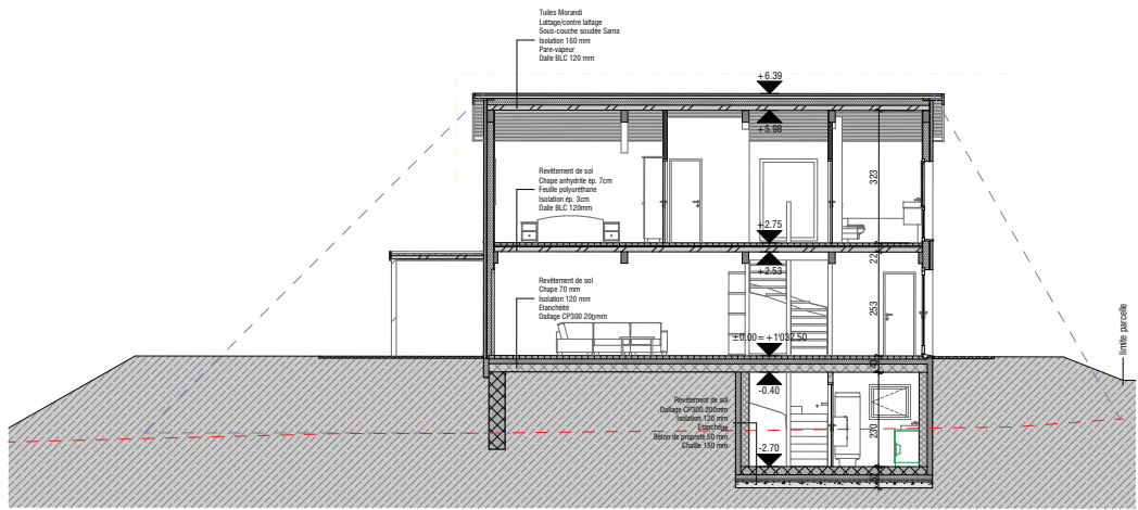
Coupe B-B
