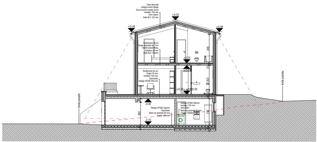
Coupe C-C
