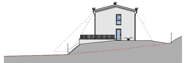
Façade Est
