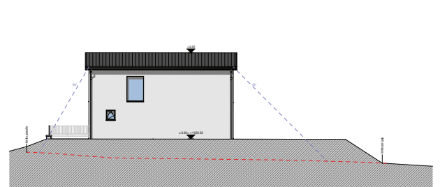
Façade Nord
